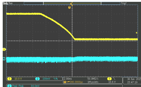
Vin=40V-12V
