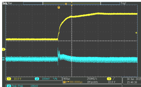
Vin=12V-40V
