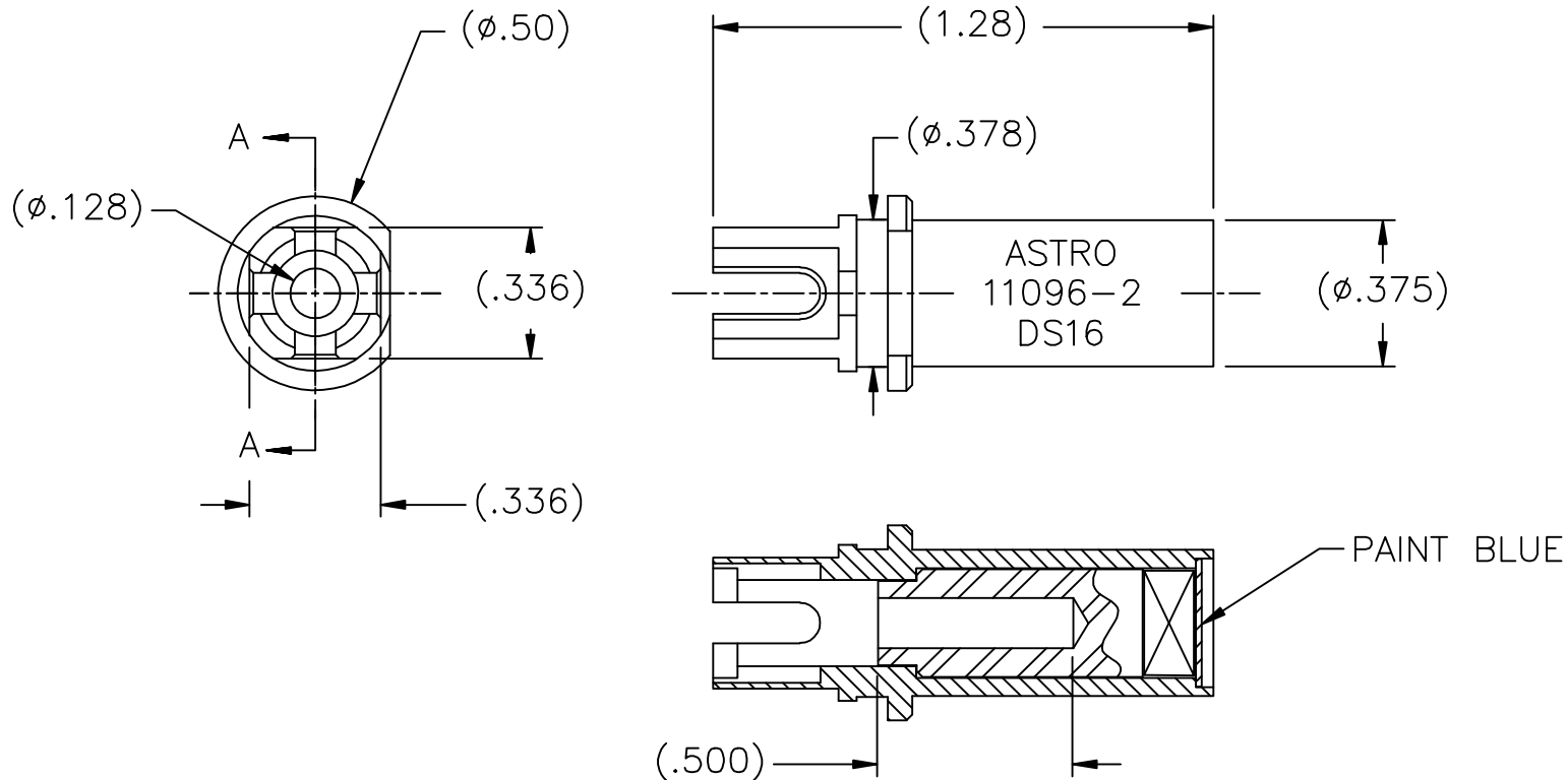
SECTION A-A
