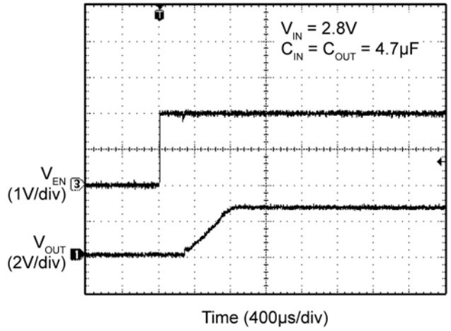
Enable Turn-On
