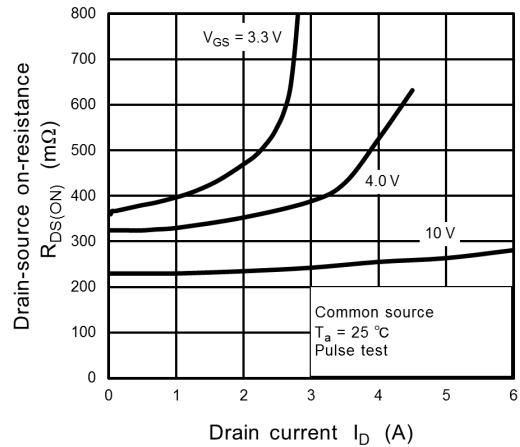
Fig. 7.6 RDS(ON) - ID
