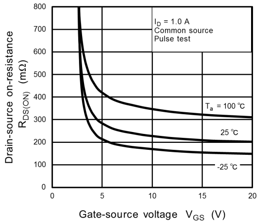
Fig. 7.5 RDS(ON) - VGS
