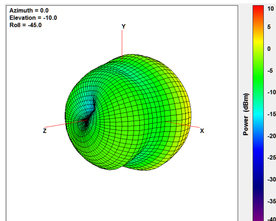
1805MHz
