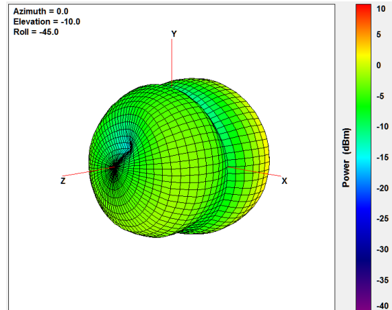
1990MHz
