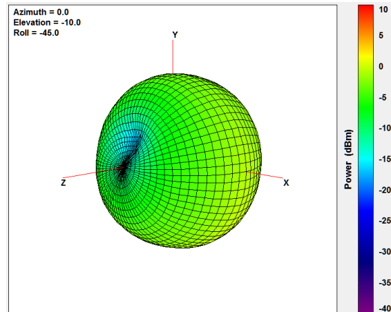
960MHz
