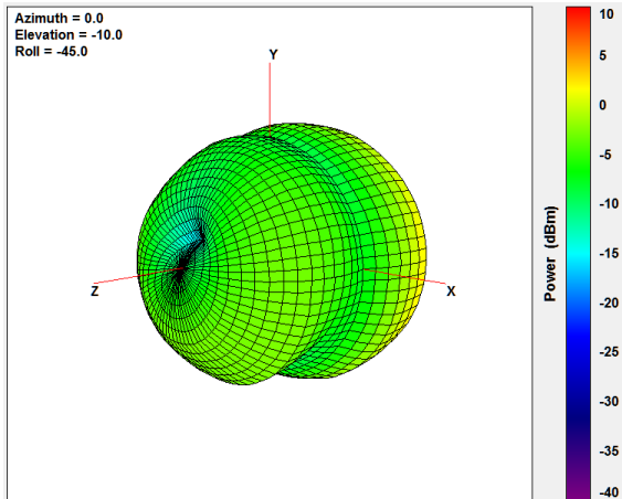
1910MHz
